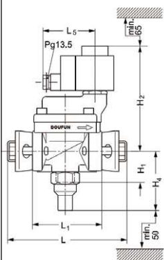
DEVSC25结构示意图
