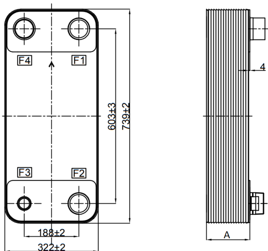
Габаритные размеры и изображение теплообменника пластинчатого паяного PHE-210
