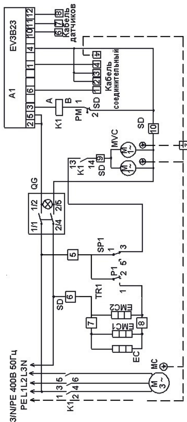
Рис.1 Питание трехфазное
